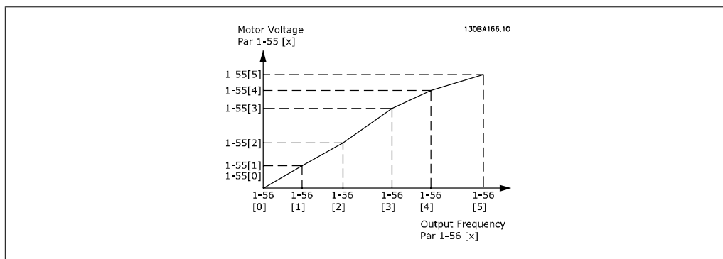
Illustration 4.1: Рис. 1 Характеристика U/f
